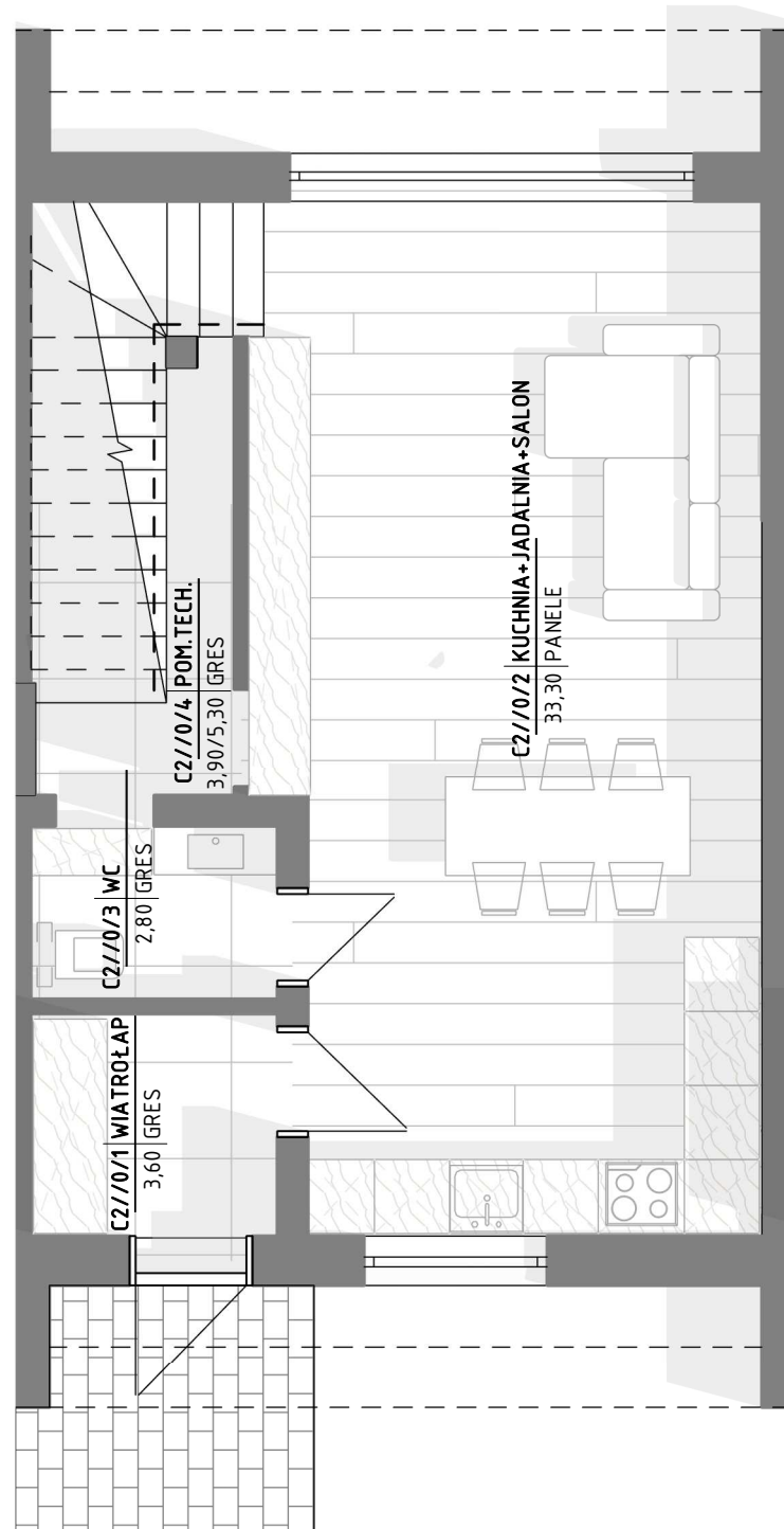
RZUT PARTERU
