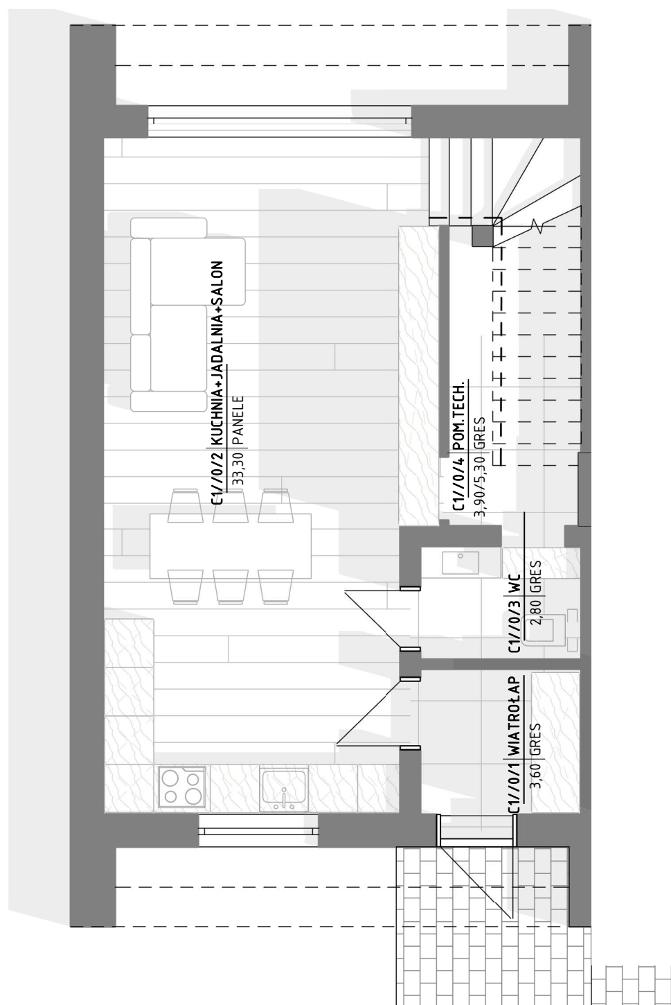
RZUT PARTERU
