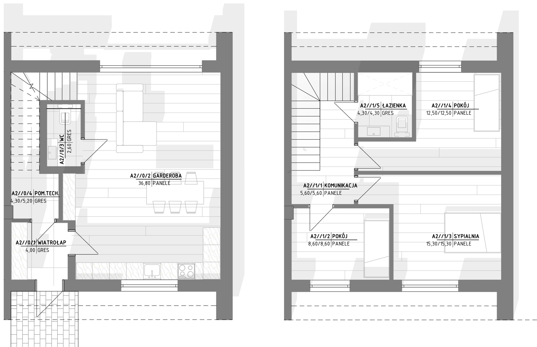
RZUT PARTERU
