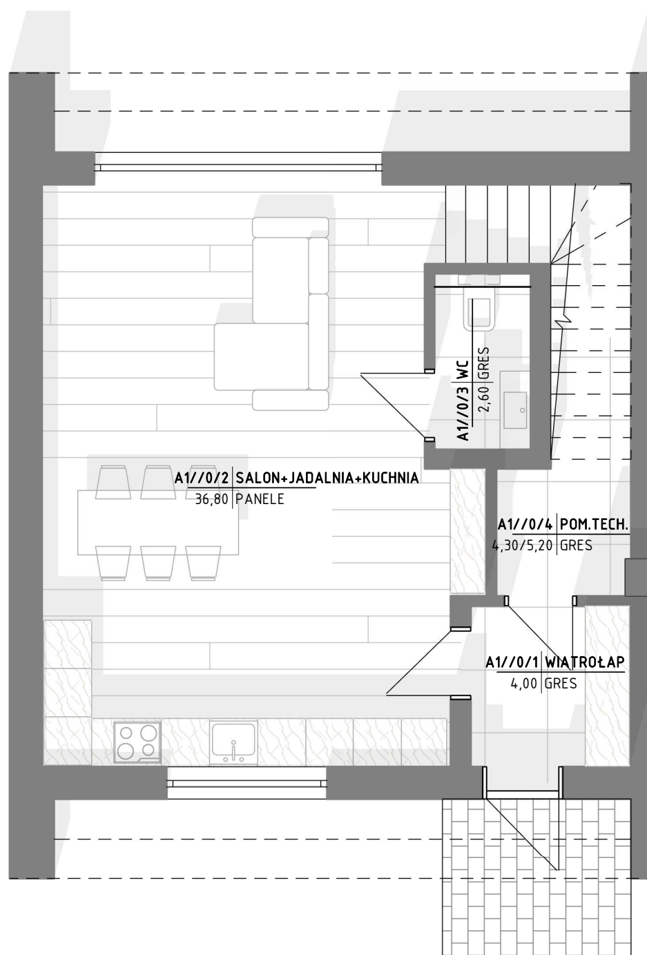
RZUT PARTERU
