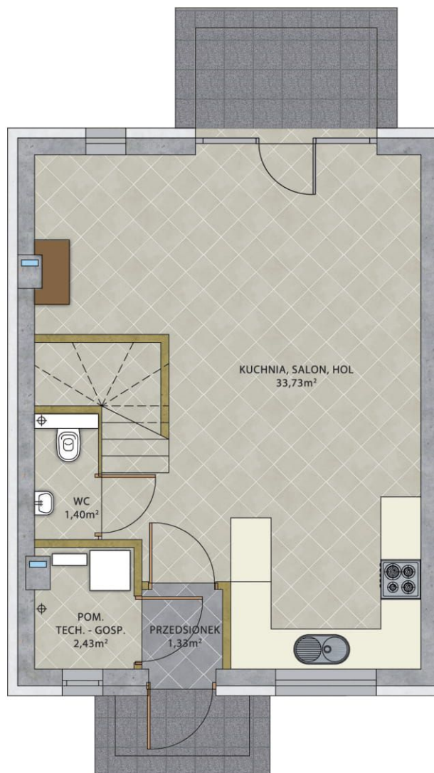
RZUT PARTERU
