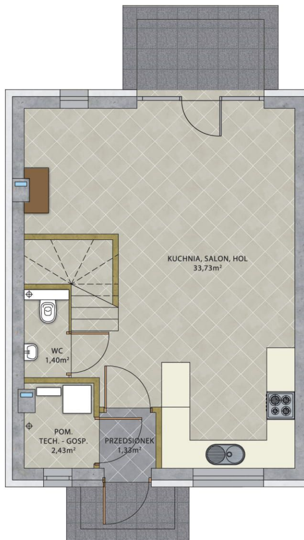
RZUT PARTERU
